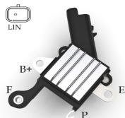
Regulador T. DENSO 104211-8210 CITROEN CACTUS
