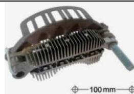
Placa Tipo MITSUBISHI 100 mm. 24v. 100 amp. 8 Diodos SCANIA P124 A4TR5191A
