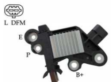
Regulador Tipo BOSCH 12v. F000BL07T1 CHEVROLET ONIX - CRUZE
