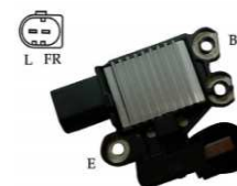
Regulador Tipo VALEO 2614390 TG12T050 12 v. 115 amp. TOYOTA COROLLA L4 1.8L 2014-2018 TOYOTA ETIOS 712910
